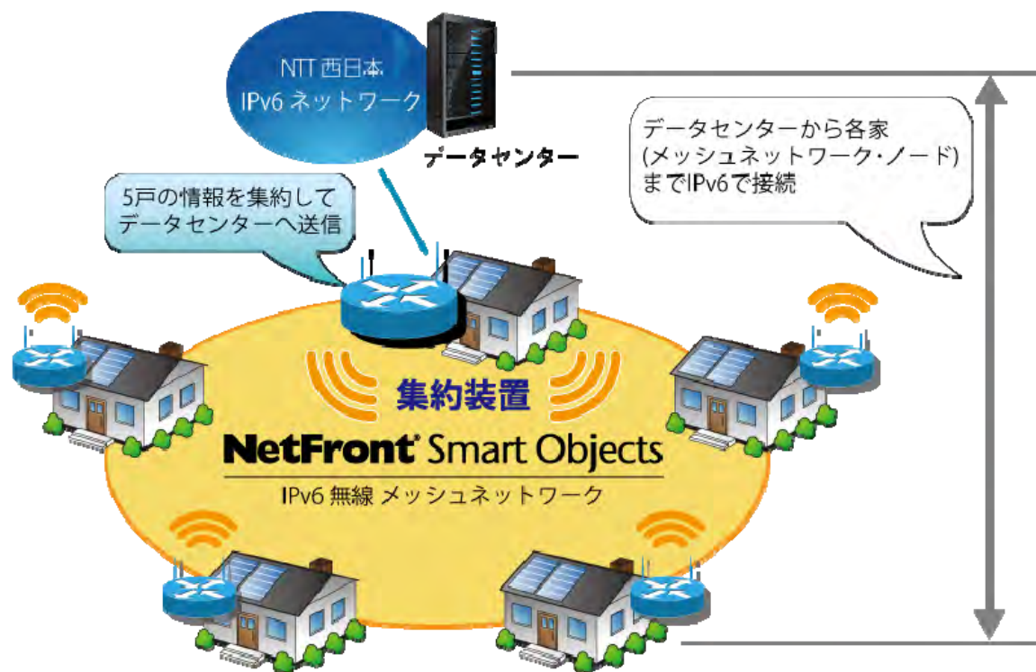
IPv6 無線メッシュネットワーク構成概要
